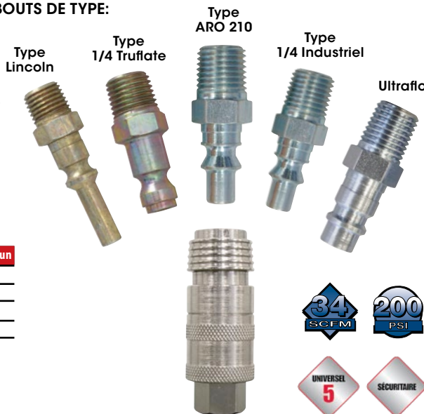
Mâle/femelle connecté
