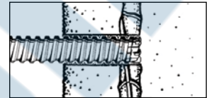
2. Utiliser un coupe-barre du même format que le foret de maçonnerie et un coupe-barre rotatif seulement pour la barre
